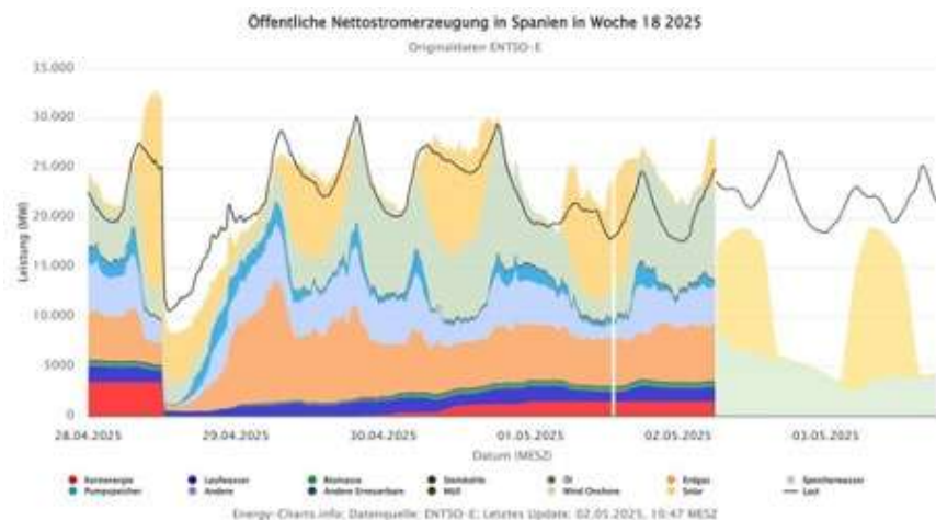
图3：2025年第18个星期，西班牙电网电力供应情况。（德国巴伐利亚州BR24截图）
